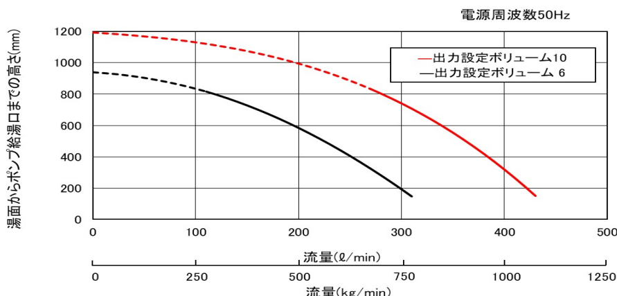
Q-H曲線(ALiP-80P及びALiP-80PH,AC4C,700℃)
