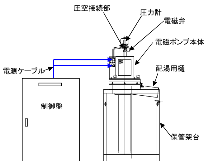
配湯用電磁ポンプ
